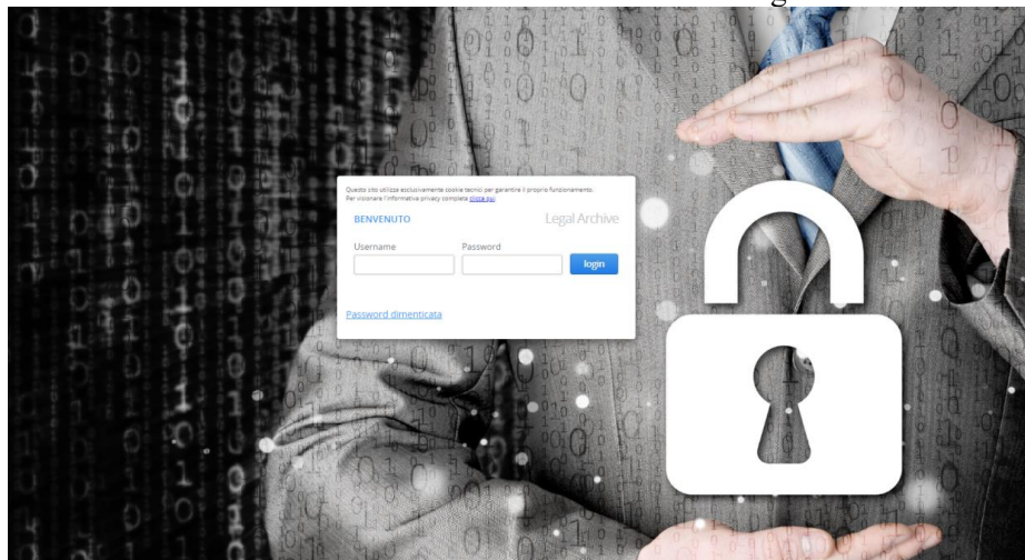
Figura 1 - LogIn
