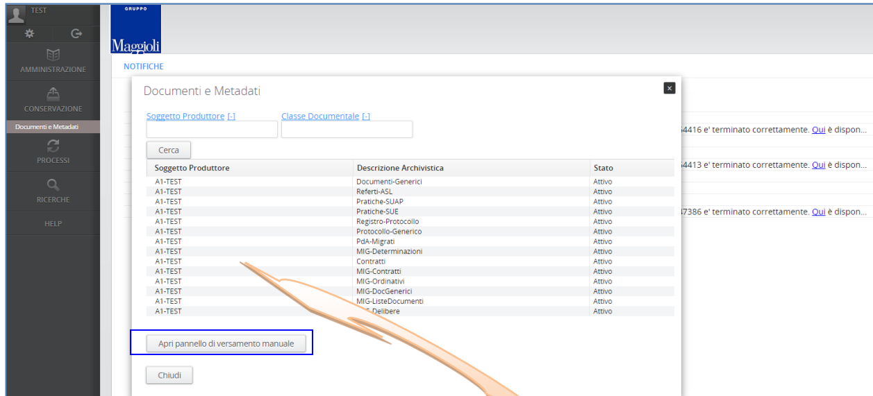
Figura 8 - Generazione SIP
